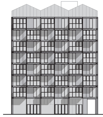
voorgevel
