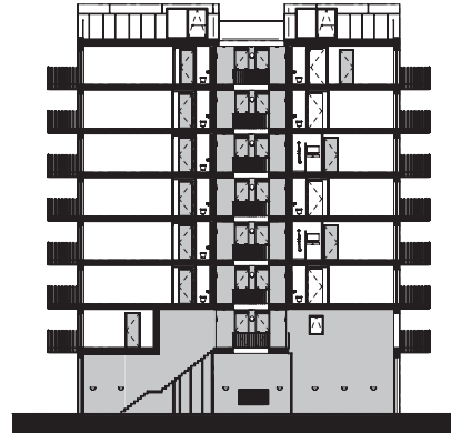
doorsnede
