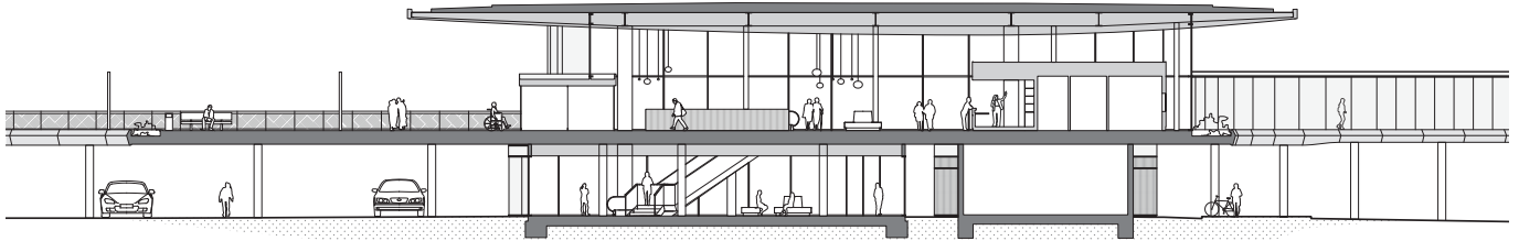
doorsnede
