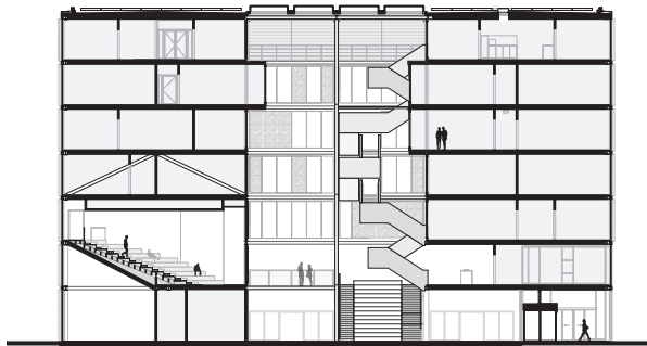
doorsnede
