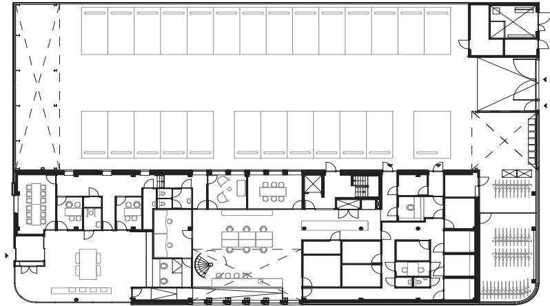
begane grond
