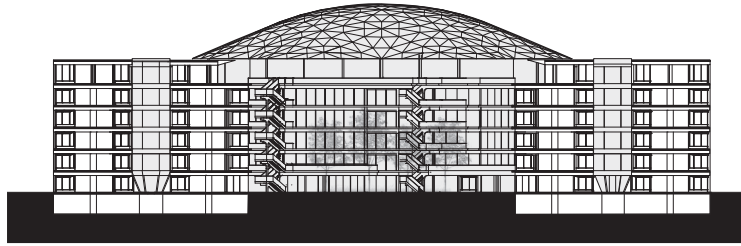
doorsnede
