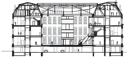
doorsnede
