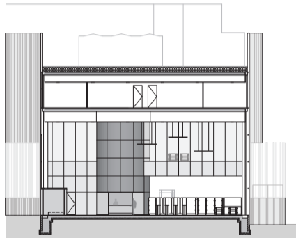
doorsnede
