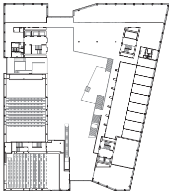
eerste verdieping
