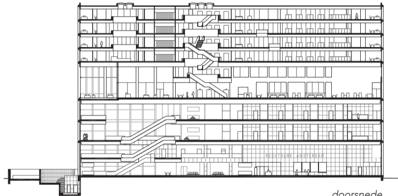
doorsnede
