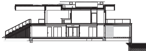
doorsnede
