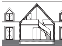
doorsnede
