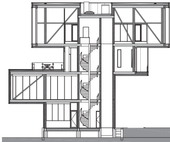
doorsnede
