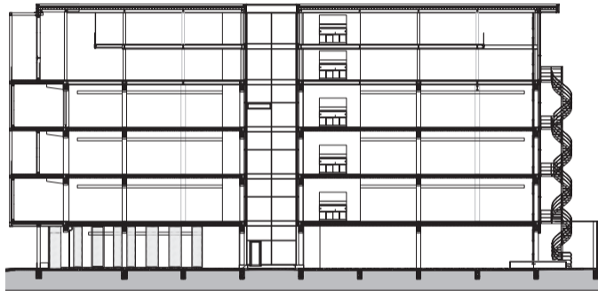
doorsnede
