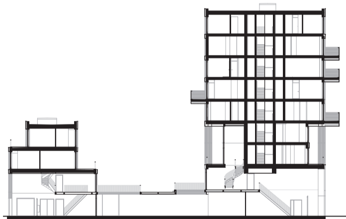
doorsnede
