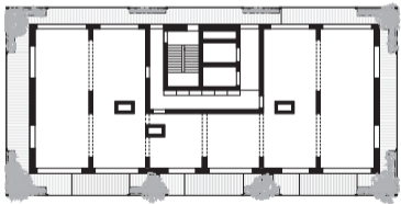
'open' plattegrond
