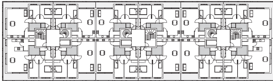
eerste verdieping
