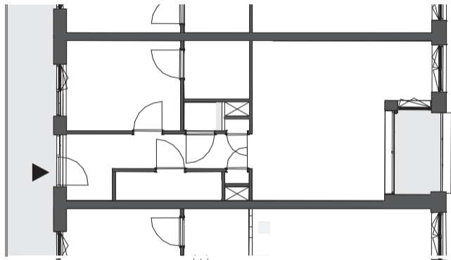
plattegrond basiswoning
