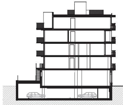
doorsnede
