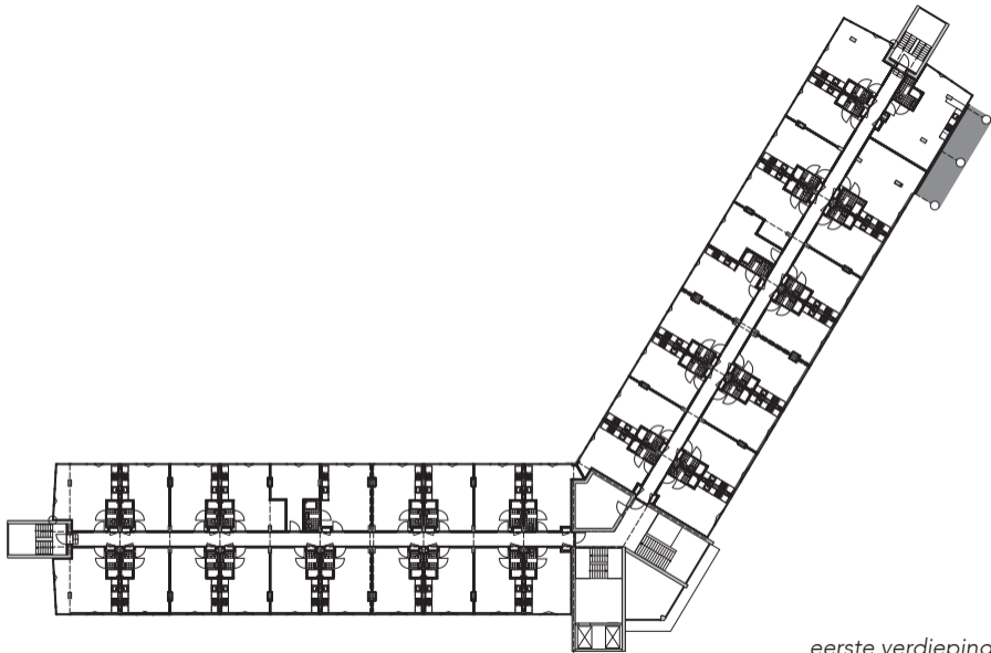
eerste verdieping
