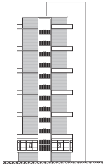
linkerzijgevel
