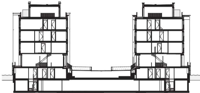
doorsnede
