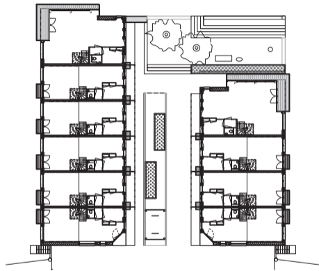
situatie met begane grond
