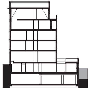
doorsnede
