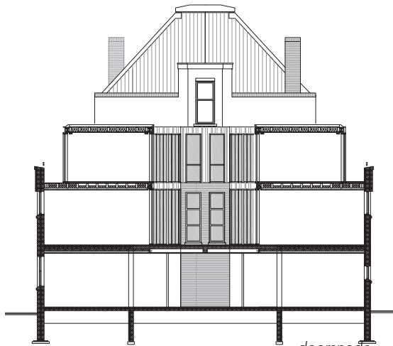
doorsnede
