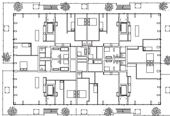
zevende verdieping
