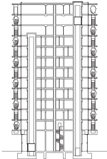
doorsnede
