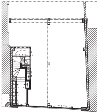
begane grond
