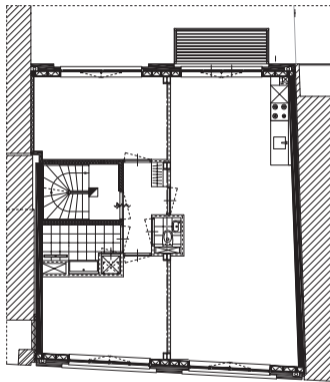
tweede verdieping
