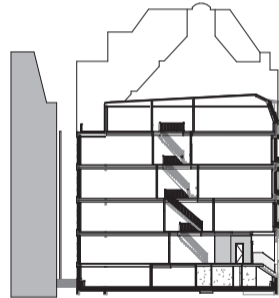
doorsnede
