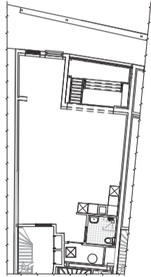
begane grond
