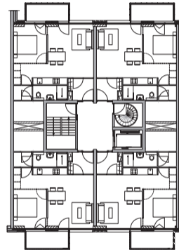
verdieping gebouw C
