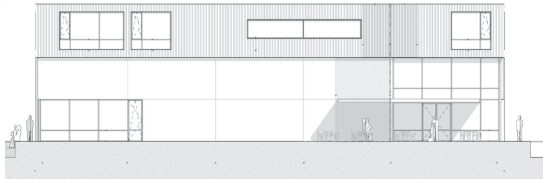
voorgevel
