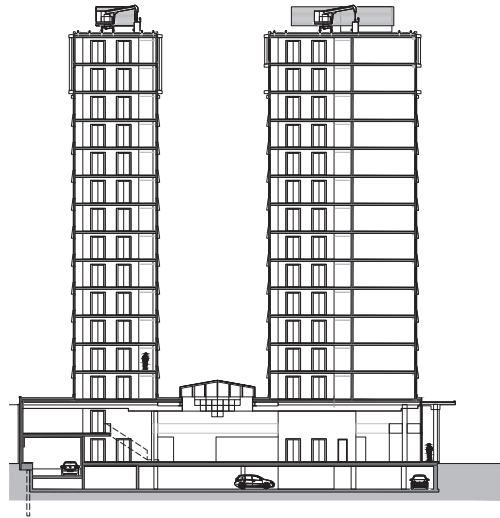
doorsnede
