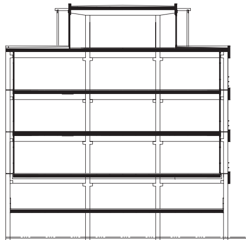
doorsnede
