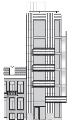
zuidoostgevel
