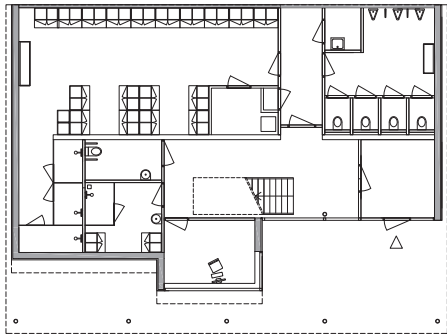
begane grond
