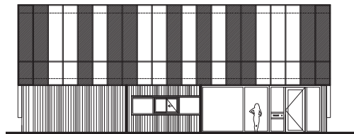
voorgevel
