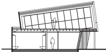
doorsnede
