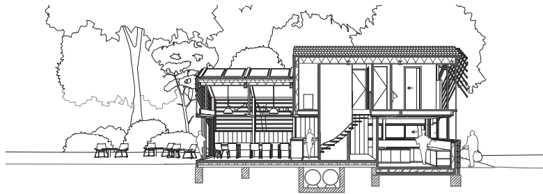
doorsnede
