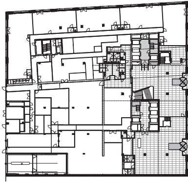
begane grond plattegrond
