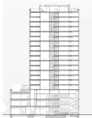
doorsnede
