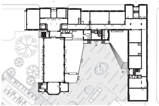
situatie met begane grond
