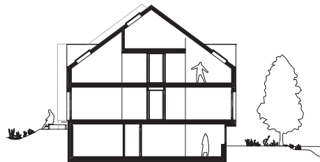
doorsnede
