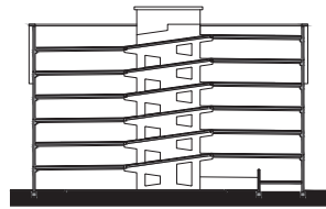
doorsnede
