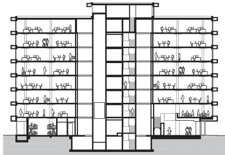
doorsnede
