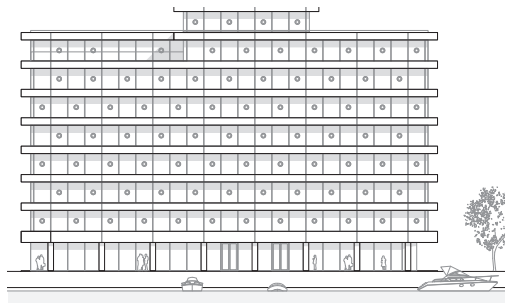
oostgevel
