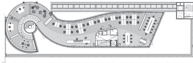
dakopbouw
