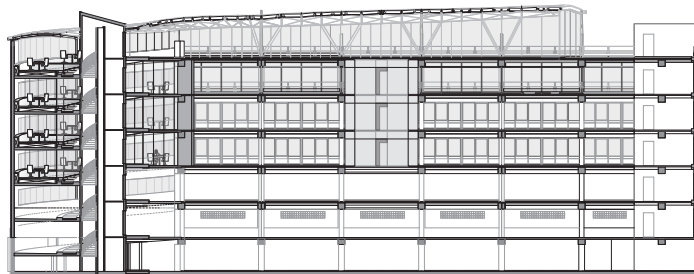
doorsnede
