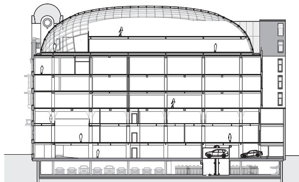
doorsnede
