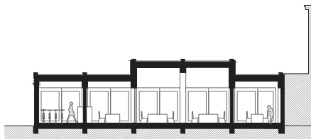
doorsnede
