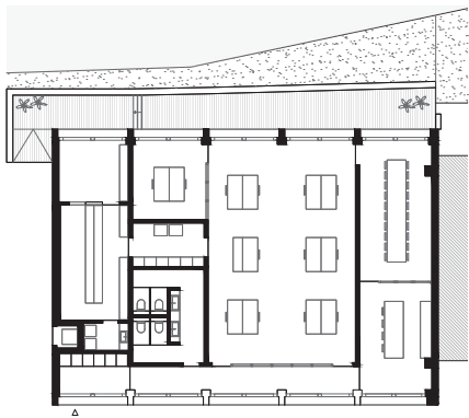
plattegrond
