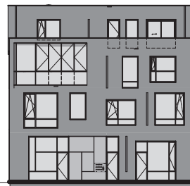
gevel voorhuis
