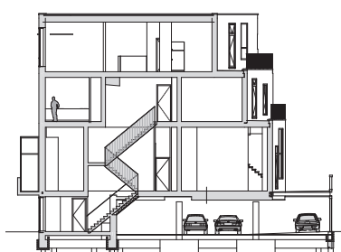
doorsnede achterhuis
