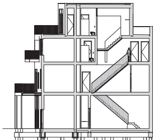
doorsnede voorhuis
