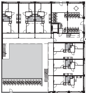
begane grond
