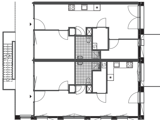
woningtype 1 en 2
