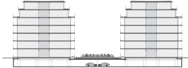
dwarsdoorsnede
