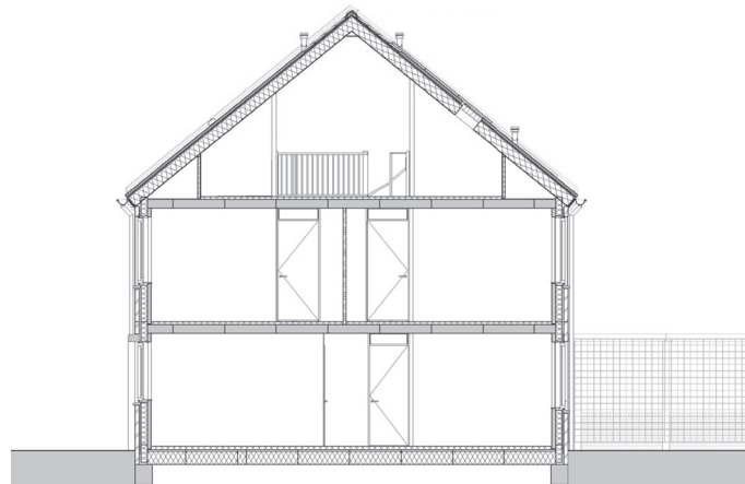
doorsnede
