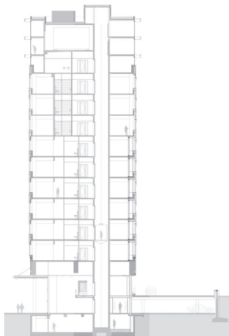
doorsnede
