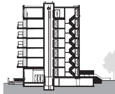
doorsnede
