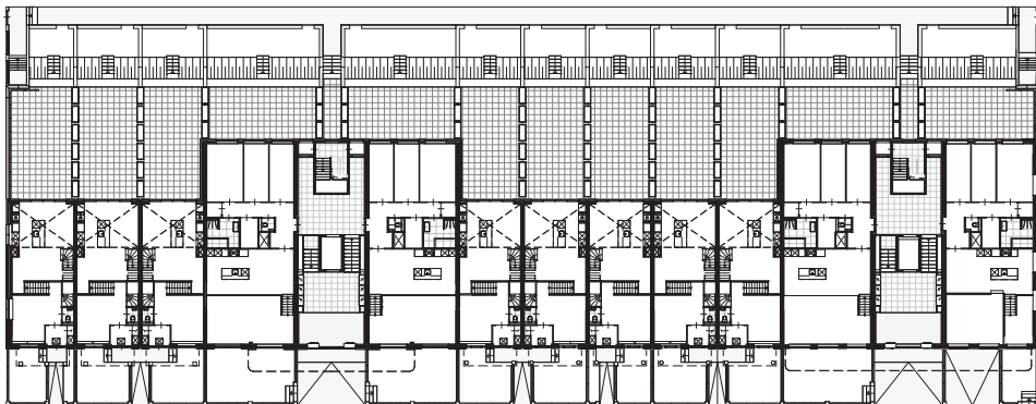
begane grond
