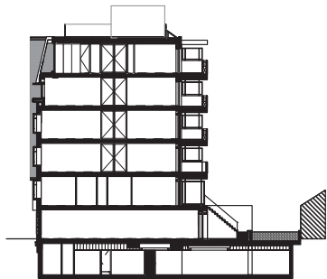
doorsnede
