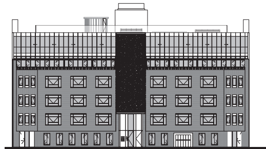
voorgevel
